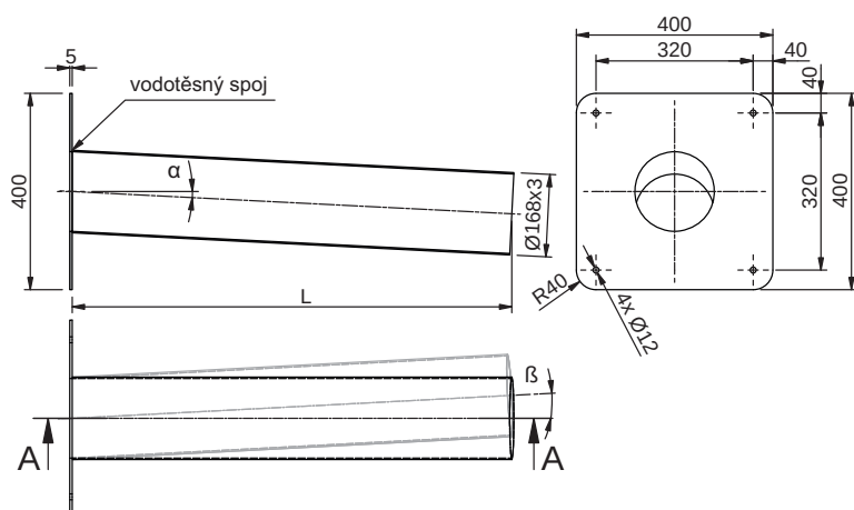
Rozměry vyústění: řez A-A
